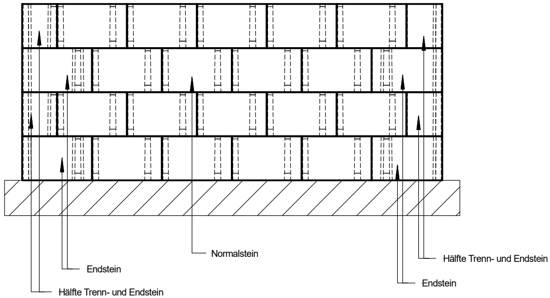
Bild 12: Ansicht
