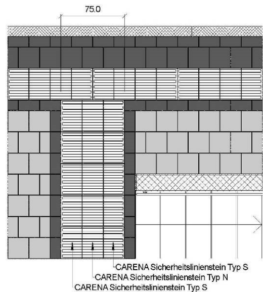
Bild 15: Anordnung von Aufmerksamkeitsfelder mit einer Breite von 75 cm mit Steinen H = 8 cm
