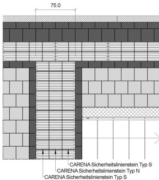
Bild 17: Anordnung von Aufmerksamkeitsfelder mit einer Breite von 75 cm mit Steinen H = 6 cm
