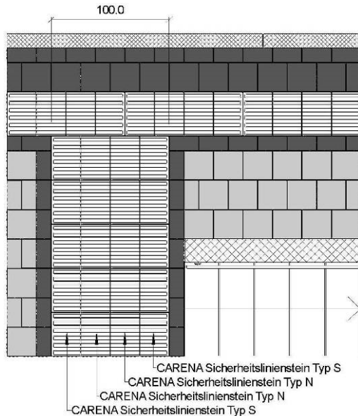
Bild 16: Anordnung von Aufmerksamkeitsfelder mit einer Breite von 100 cm mit Steinen H = 8 cm
