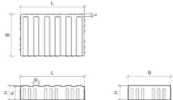
Bild 6: CARENA® Sicherheitslinienstein Typ S; H 8 cm
