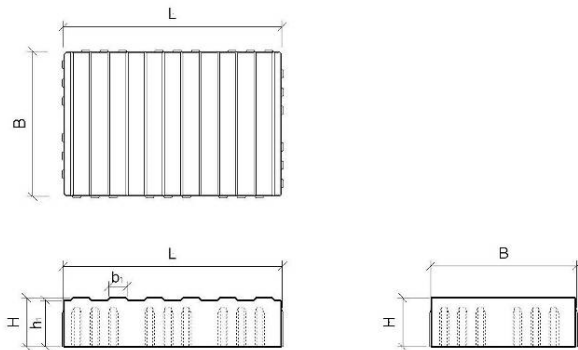
Bild 5: CARENA® Sicherheitslinienstein Typ N; H 8 cm
