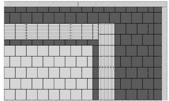
Bild 14: Anordnung beim Ende einer Perronanlage
