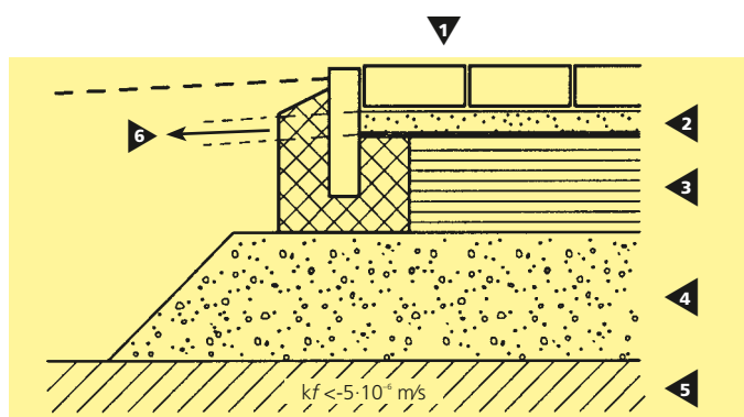
Wasserabfuhr durch die Pflasterbettung Darstellung 23
