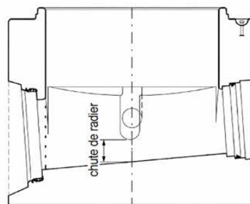
Illustration 19 : pour les petits diamètres nominaux, il est recommandé de prévoir un dénivelé dans les fonds de chambre spéciaux CENTUB®
