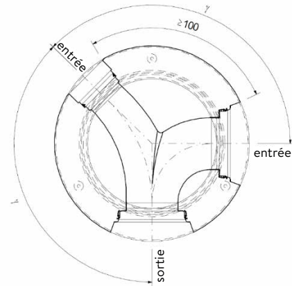
Illustration 15 : angles intermédiaires dans les fonds de chambre spéciaux CENTUB®
