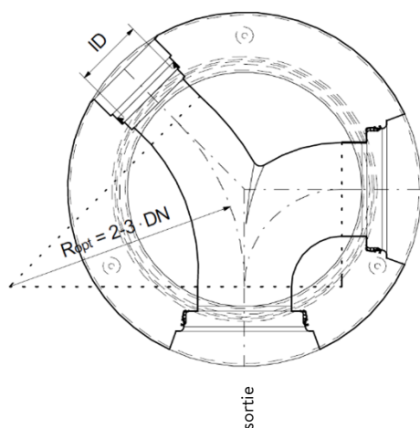
Illustration 22 : rayon de courbure optimal pour les fonds de chambre spéciaux CENTUB®
