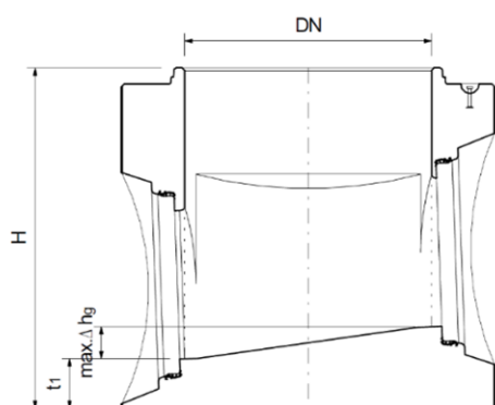
Illustration 16 : différence de hauteur pour les fonds de chambre spéciaux CENTUB®
