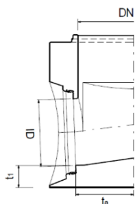
Illustration 12 : raccordement avec joint intégré dans la paroi du regard
