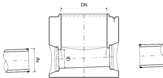
Illustration 6 : raccordement avec tuyaux en grès de type H avec pente J \leq 150\text{‰}
