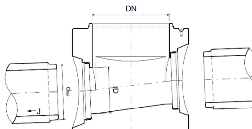
Illustration 2 : raccordement par tuyaux en béton armé CENTUB® Röser de pente J \leq 150\text{‰}
