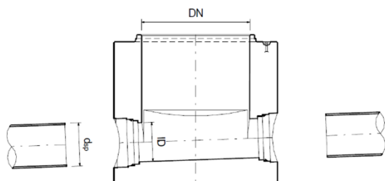
Illustration 9 : raccordement avec tuyaux en polyéthylène avec pente J ≤ 150‰
