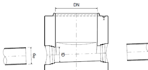
Illustration 10 : raccordement avec tuyaux en polychlorure de vinyle avec pente J ≤ 150‰
