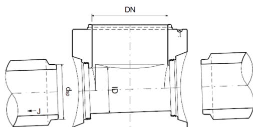
Illustration 3 : raccordement par tuyaux en béton armé ROBUST® Röser avec pente J ≤ 150‰
