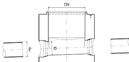
Illustration 8 : raccordement avec tuyaux en polypropylène avec pente J \leq 150\text{‰}
