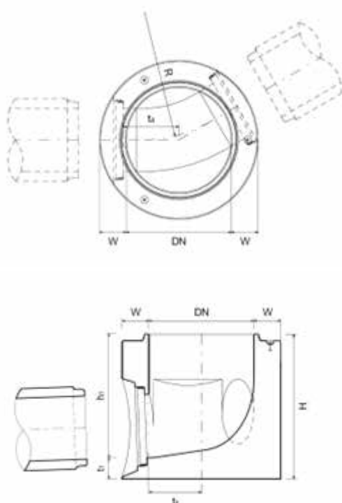
Illustration 1 : fond de chambre spécial coulé CENTUB®
