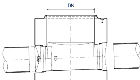
Illustration 7 : raccordement avec tuyaux en fonte ductile avec pente J \leq 150\text{‰}
