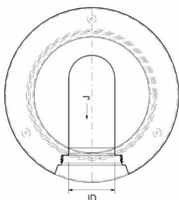
Illustration 17 : fond de chambre spécial CENTUB® sans entrée
