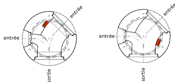
Niche marche-pieds sortie gauche Niche marche-pieds sortie droite
