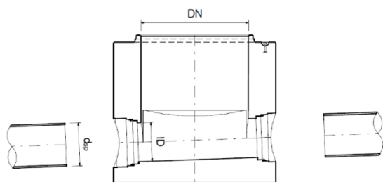
Illustration 11 : raccordement avec tuyaux en polyester insaturé renforcé de fibres de verre avec pente J ≤ 150‰
