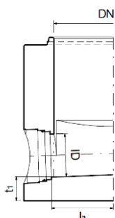
Illustration 13 : raccordement avec joint libre dans la paroi du regard
