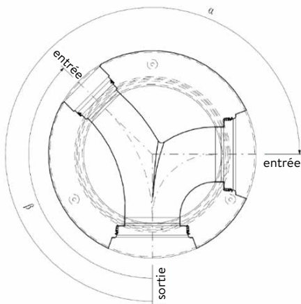
Illustration 14 : angles de raccordement pour fond de chambre spécial CENTUB®
