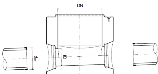
Illustration 5 : raccordement avec tuyaux en grès de type N avec pente J \leq 150\text{‰}
