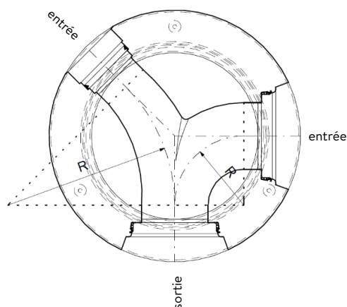
Illustration 18 : entrée et arrivée dans un fond de chambre spécial CENTUB®
