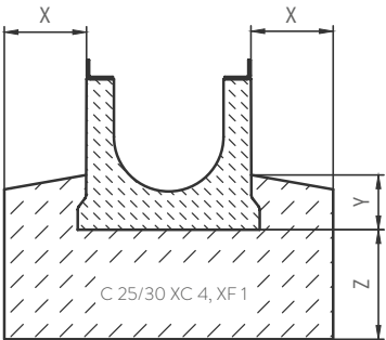
Montage suivant catalogue des structures types de chaussées avec de couches de fondation anti-gel (composition libre)
