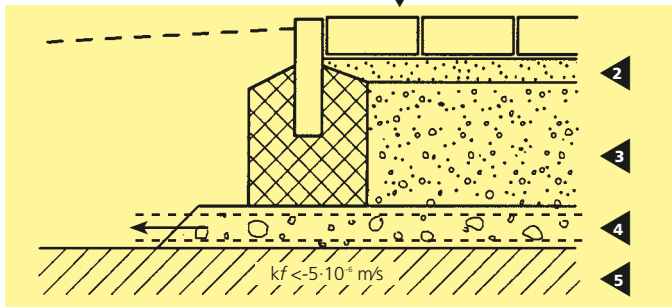
Wasserableitung oberhalb des Planums bei nicht ausreichend versickerungsfähigem Untergrund Darstellung 22
