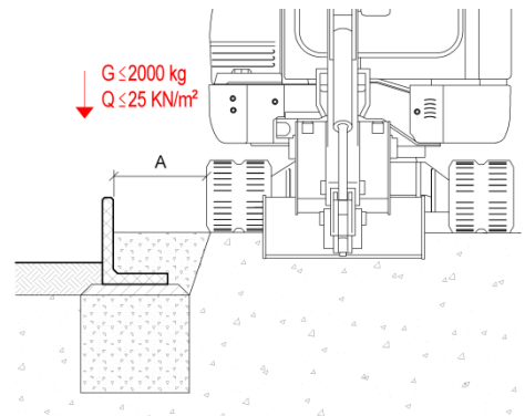
Bild 11: Lastfall G
