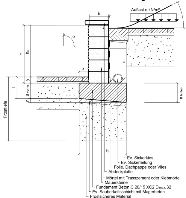
Bild46: Vertikaler Maueraufbau
