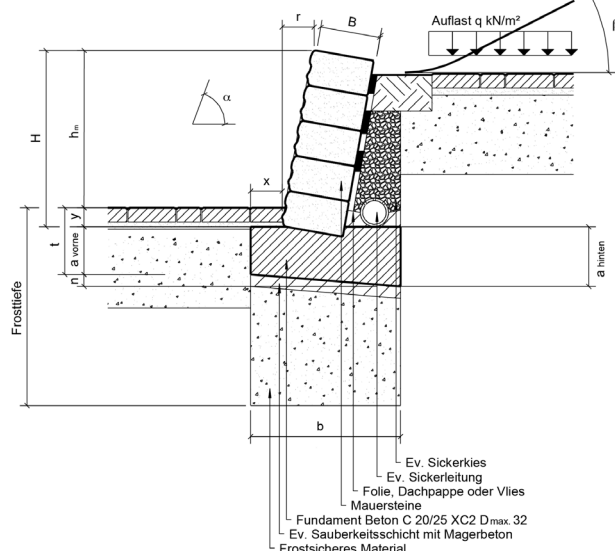
Lastfall A: Horizontale Hinterfüllung ohne zusätzliche Auflast Lastfall B: Horizontale Hinterfüllung mit zusätzlicher Auflast 5 kN/m 2 Lastfall C: Horizontale Hinterfüllung mit zusätzlicher Auflast 10 kN/m 2 Lastfall D: Böschungsneigung oberhalb der Hangsicherung 1:3, \beta 18° Lastfall E: Böschungsneigung oberhalb der Hangsicherung 1:2, \beta 27°
