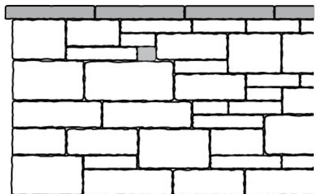
Mauertyp 20, Mauerhöhe 0.98 m
