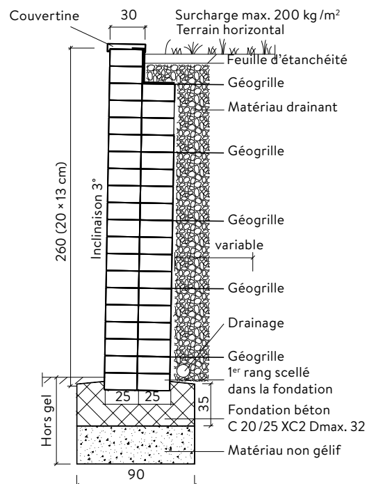
Exemple de réalisation d'un mur avec une armature en géogrid, épaisseur = 50 cm
