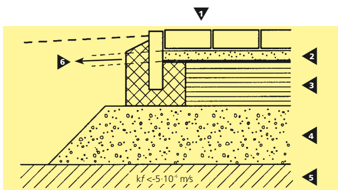
Wasserableitung durch die Pflasterbettung
