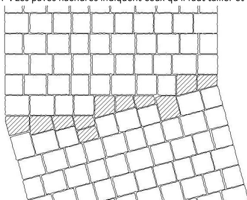
Schéma de pose possible de changement de direction avec les pavés FRIEDA®. Les pavés hachurés indiquent ceux qu'il faut tailler et ajuster.
