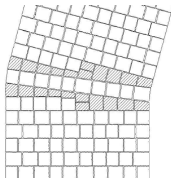
Schéma de pose possible de changement de direction avec les pavés FRIEDA®. Les pavés hachurés indiquent ceux qu'il faut tailler et ajuster.
