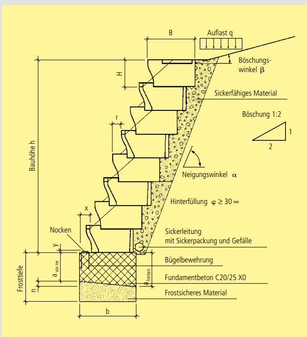
Böschungselemente Aufbau
