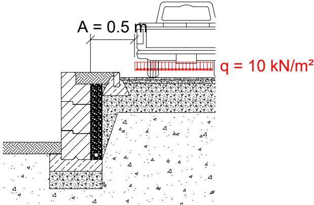
Illustration 6 : cas de charge C
