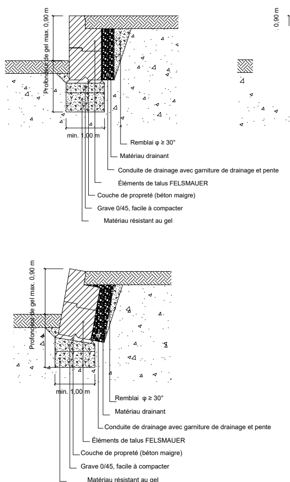
Illustration 10 : représentation schématique de la pose sans semelle filante
