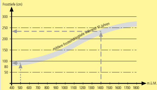
Mittlere Frostdringtiefe während 10 Jahren im Kiesmaterial.
