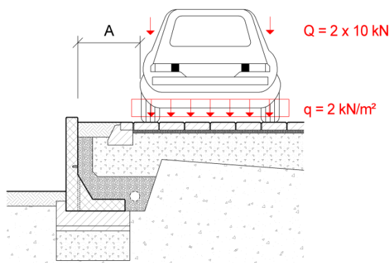
Bild 9: Lastfall B2
