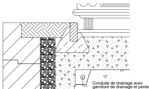
Illustration 20 : drainage supplémentaire
