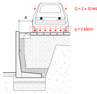
Bild 12: Lastfall B2
