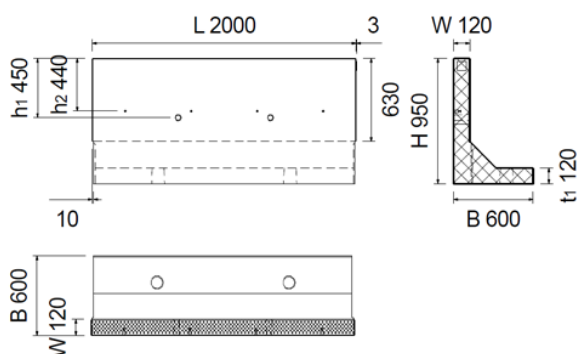
Illustration 5 : Bordures de quai de type 5
