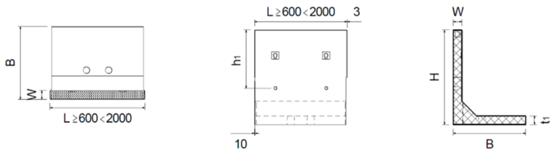
Illustration 9 : Pièce d'ajustement
