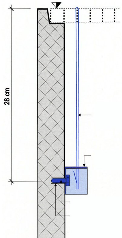
Bild 15: Einbruchsicherung
