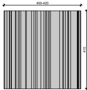
Schnitt 1-1 1:10
