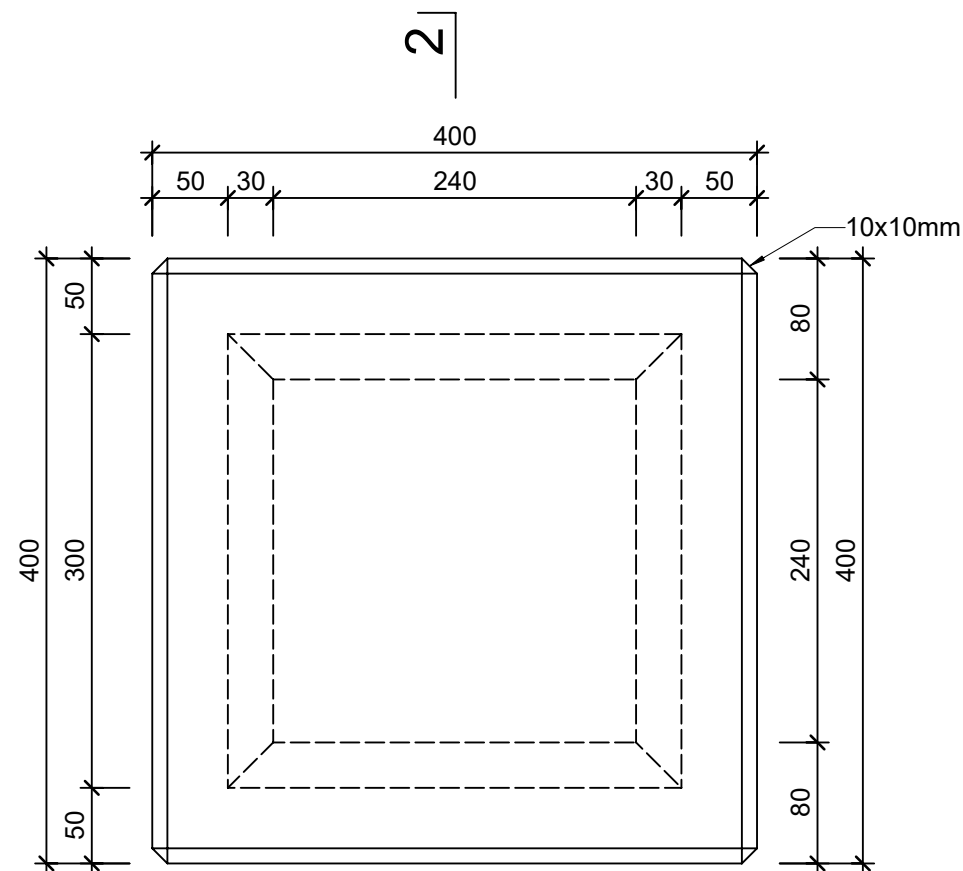
Grundriss, 1:5
