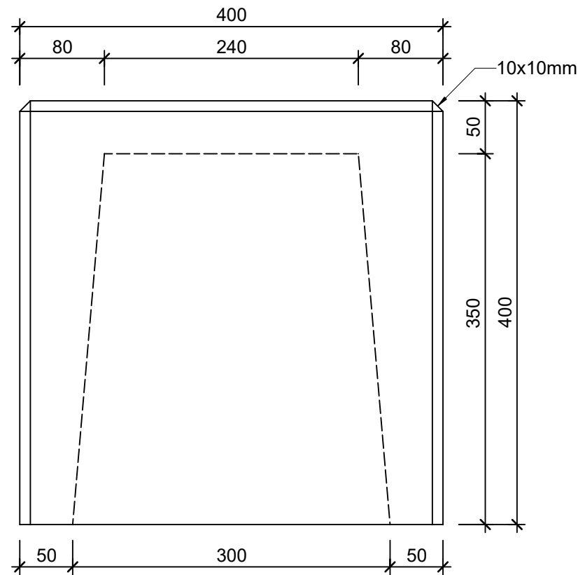
Ansicht 1-1, 1:5
