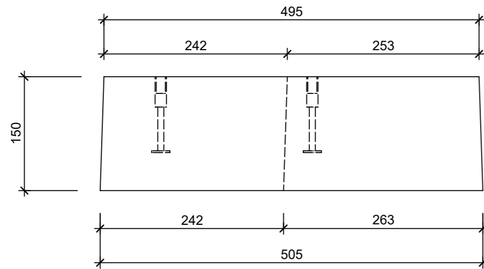
Grundriss, 1:5
