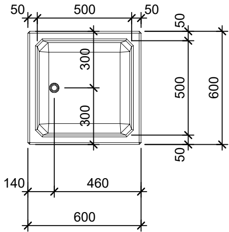
Grundriss 1:20
