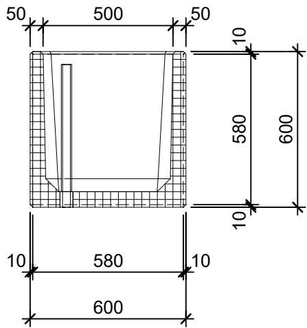
Schnitt 1-1 1:20
