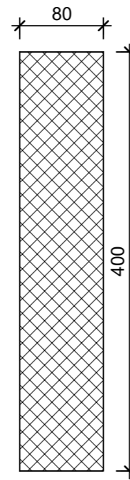
Schnitt 2-2, 1:5
