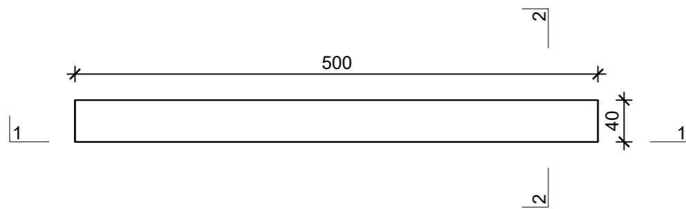
Grundriss, 1:5
