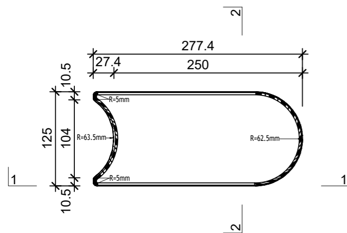
Grundriss, 1:5
