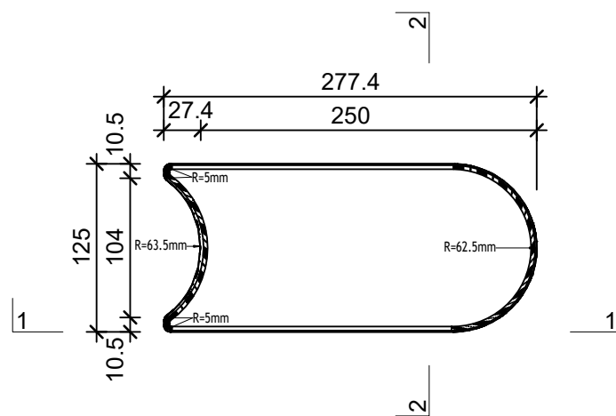
Grundriss, 1:5
