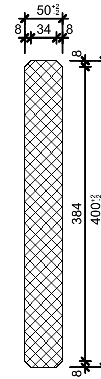
Schnitt 2-2, 1:5
