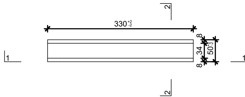
Grundriss, 1:5
