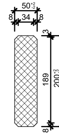
Schnitt 2-2, 1:5
