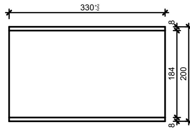
Schnitt 1-1, 1:5
