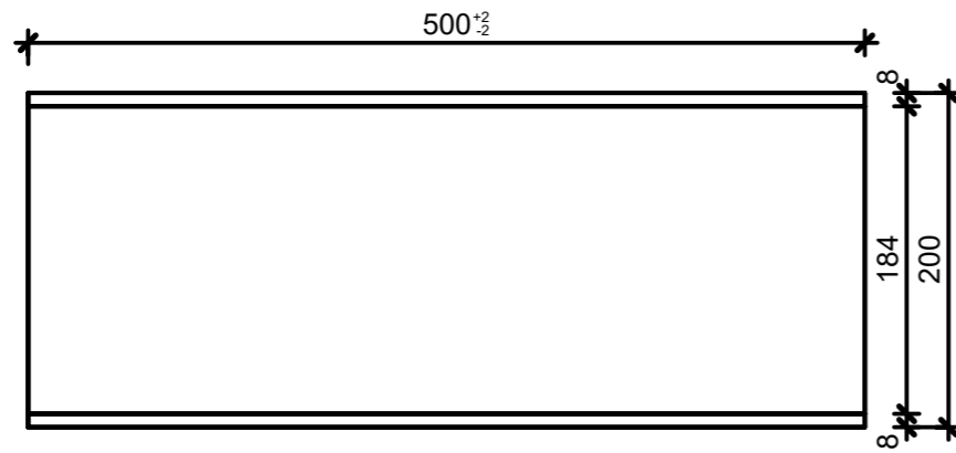
Schnitt 1-1, 1:5
