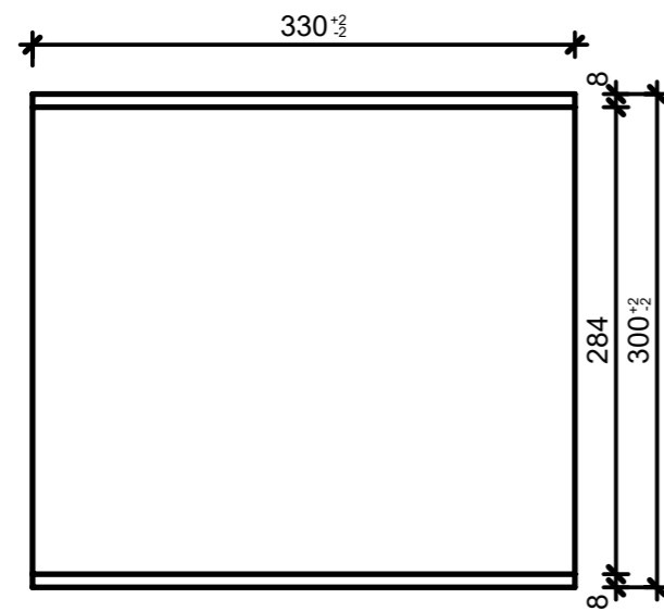
Schnitt 1-1, 1:5
