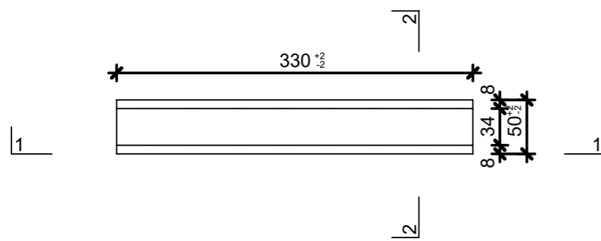
Grundriss, 1:5
