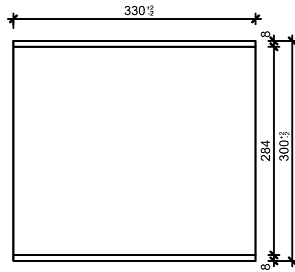
Schnitt 1-1, 1:5
