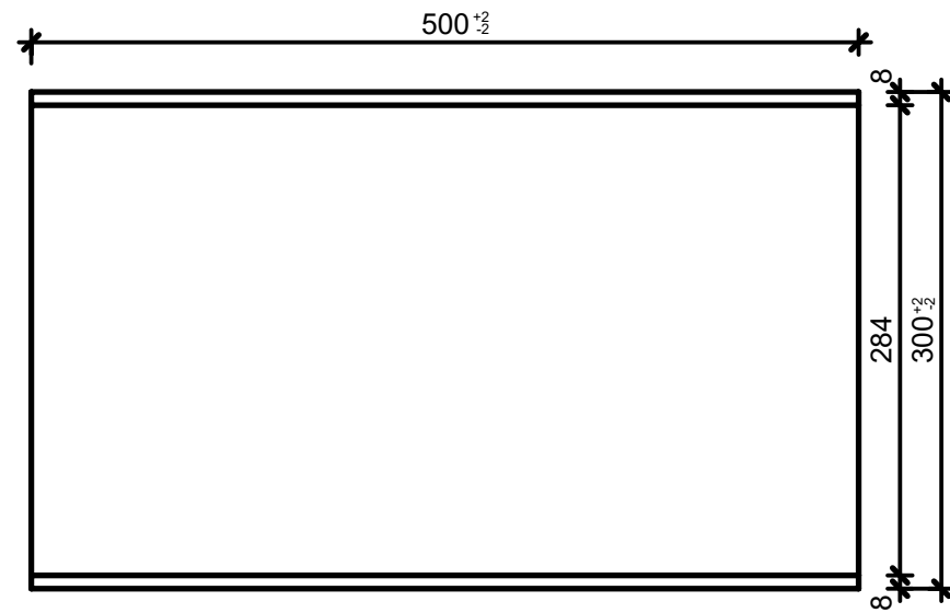
Schnitt 1-1, 1:5
