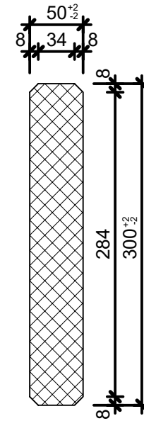
Schnitt 2-2, 1:5
