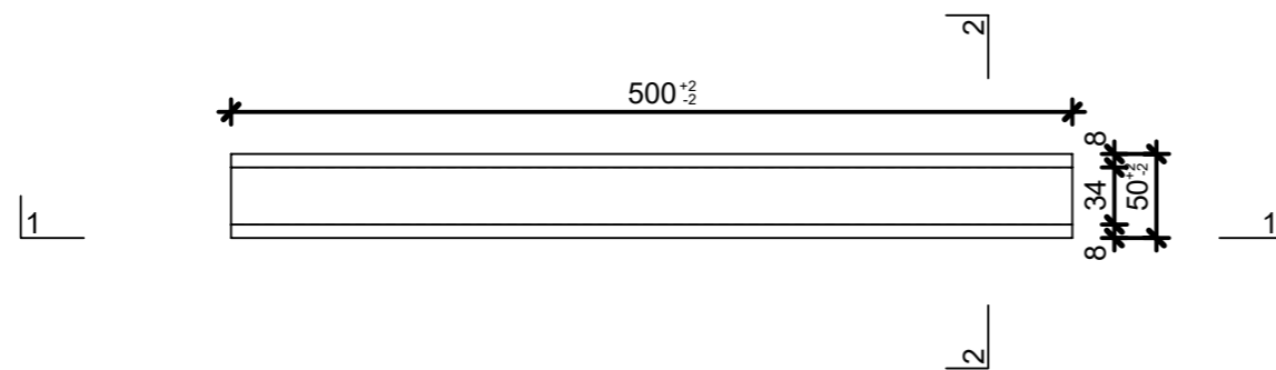
Grundriss, 1:5
