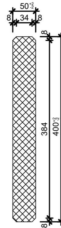
Schnitt 2-2, 1:5
