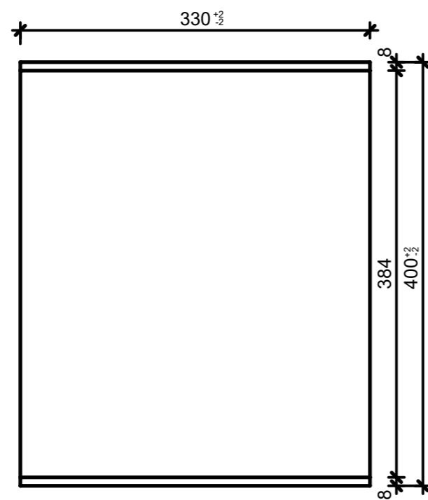
Schnitt 1-1, 1:5
