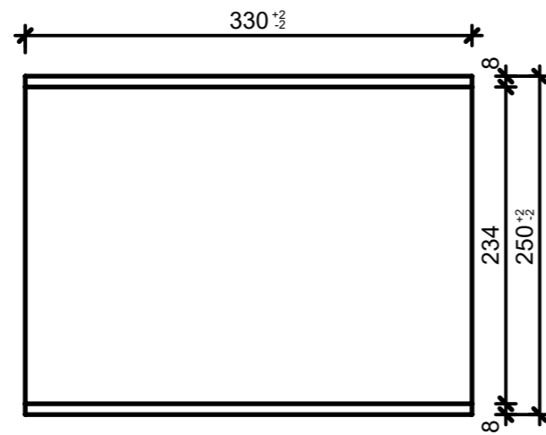
Schnitt 1-1, 1:5
