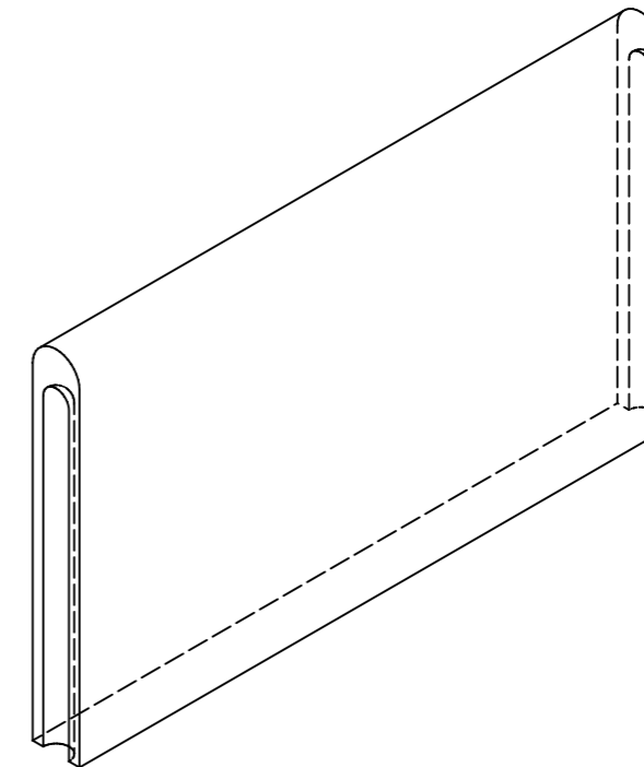
Isometrie, 1:5
