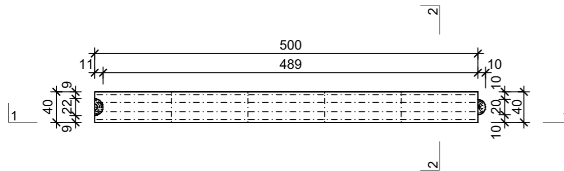
Grundriss, 1:5
