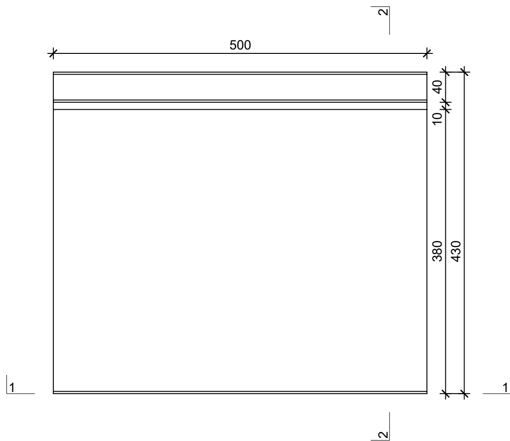
Grundriss, 1:5
