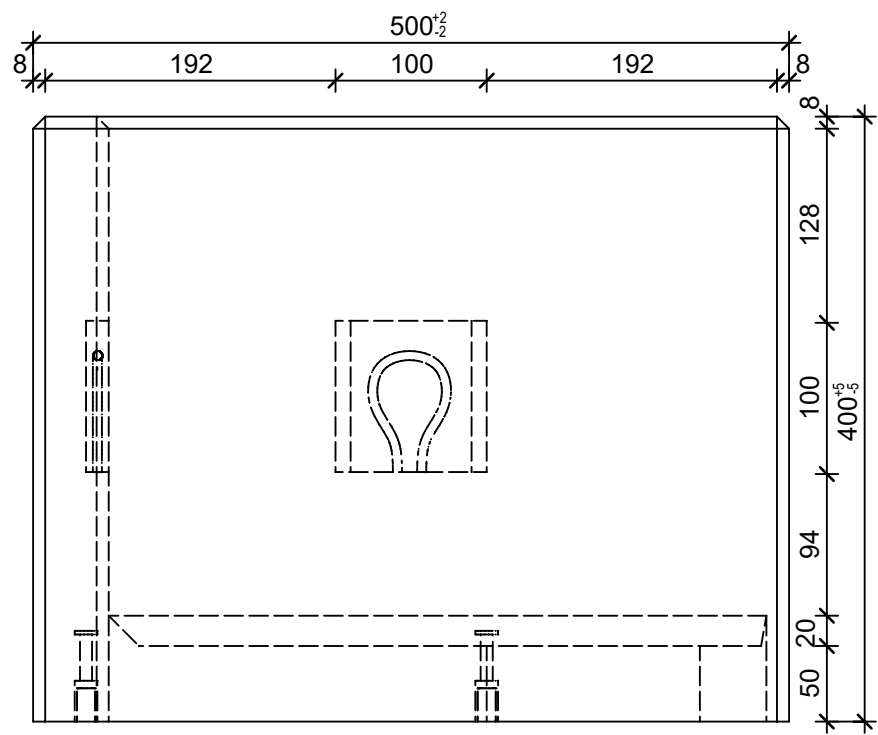
Schnitt 1-1, 1:5
