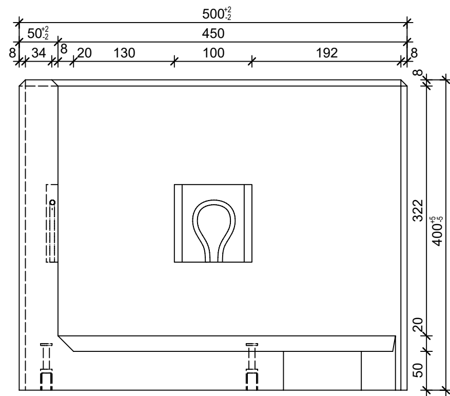
Schnitt 2-2, 1:5
