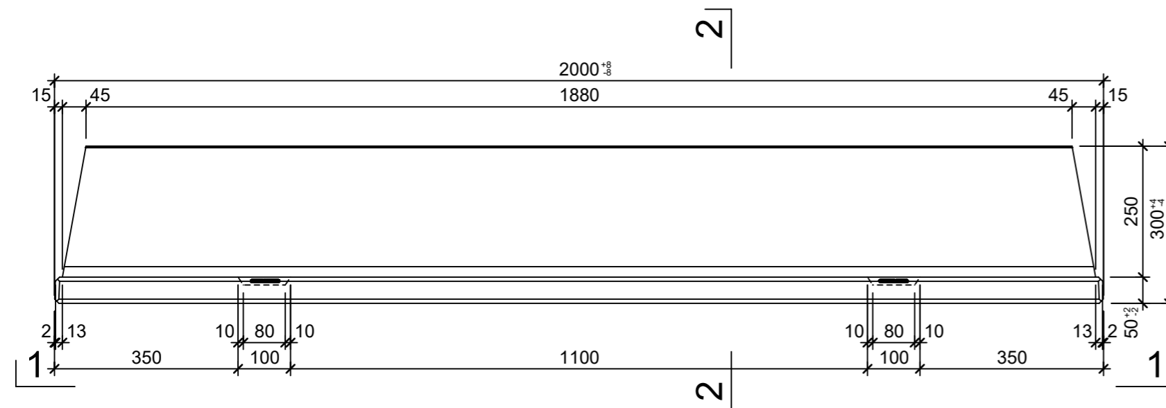
Grundriss 1:10
