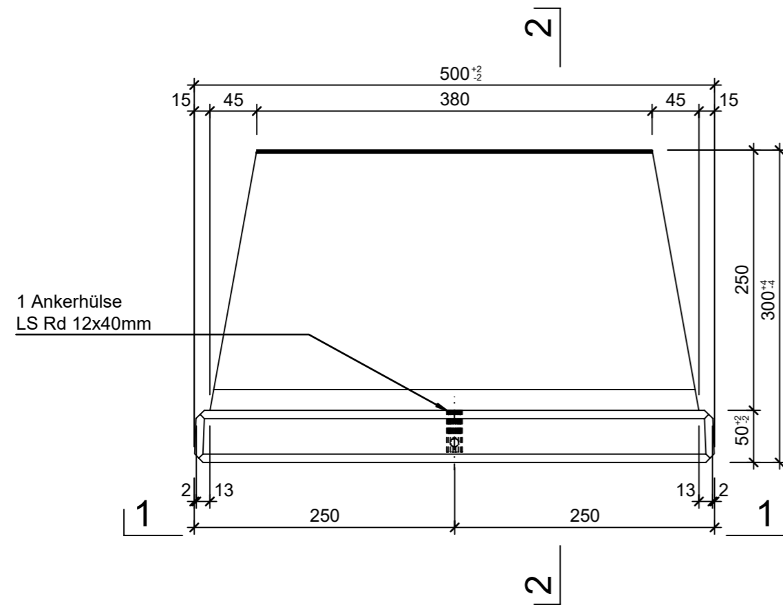
Grundriss 1:5
