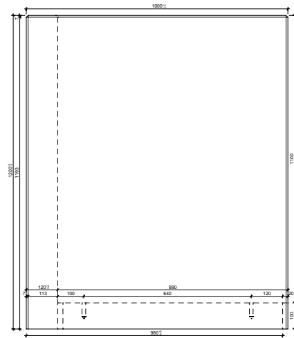
Grundriss, 1:20
