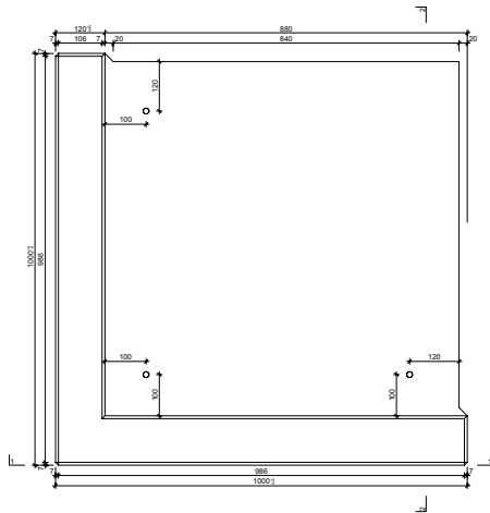
Grundriss, 1:20
