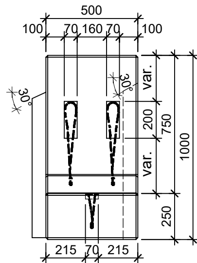
Schnitt 1-1, 1:20
