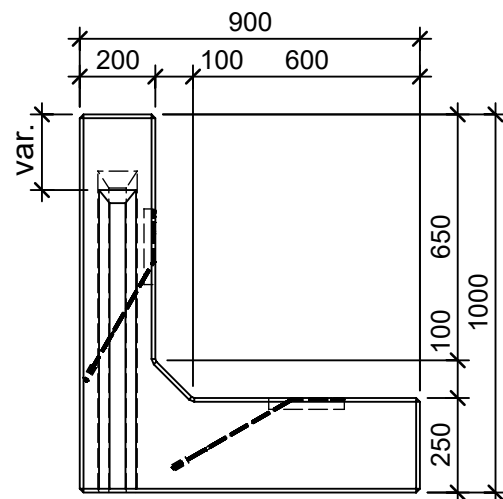
Schnitt 2-2, 1:20
