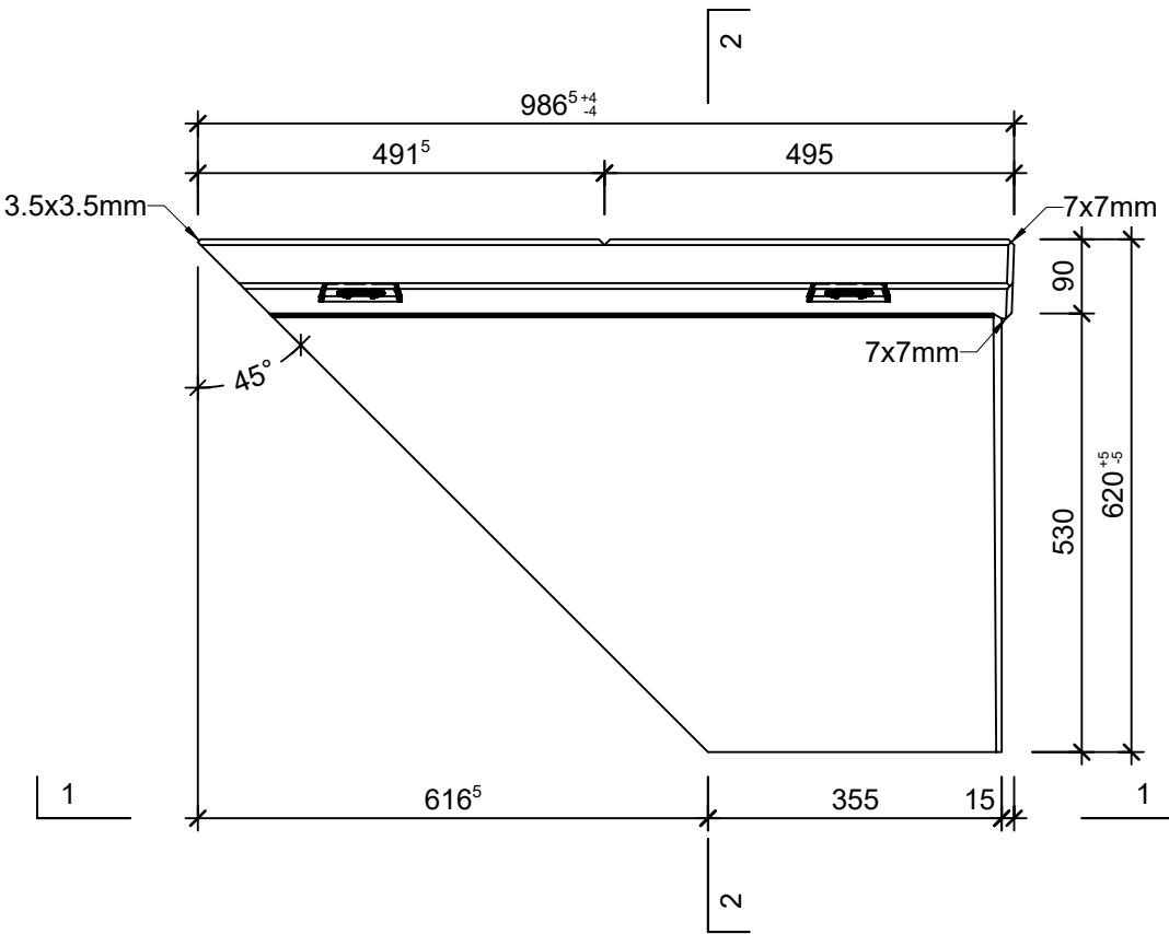
Grundriss, 1:10
