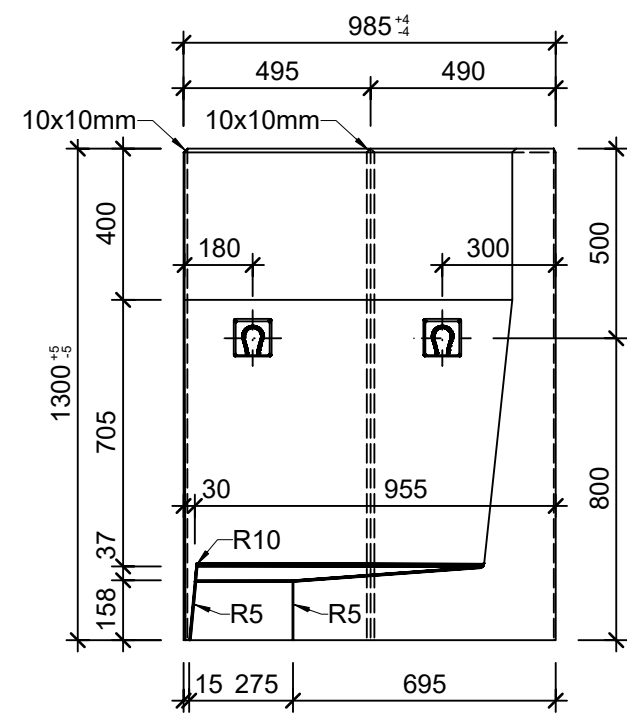
Ansicht 1-1, 1:20
