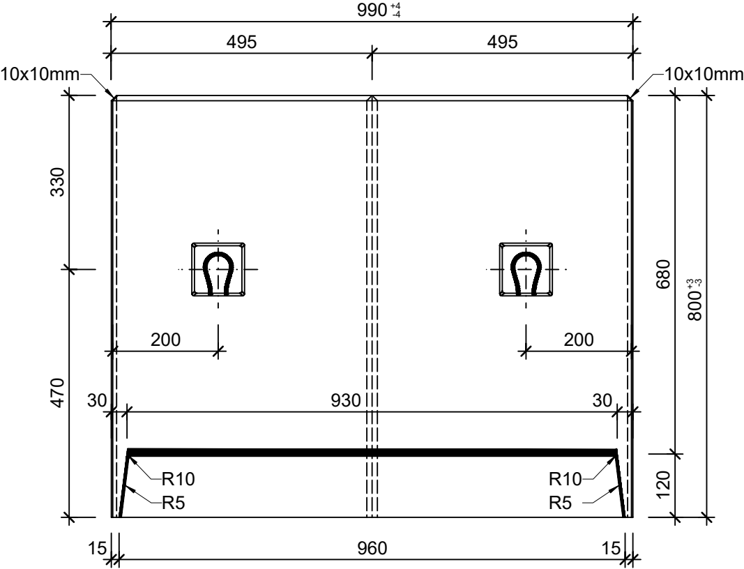
Ansicht 1-1, 1:10
