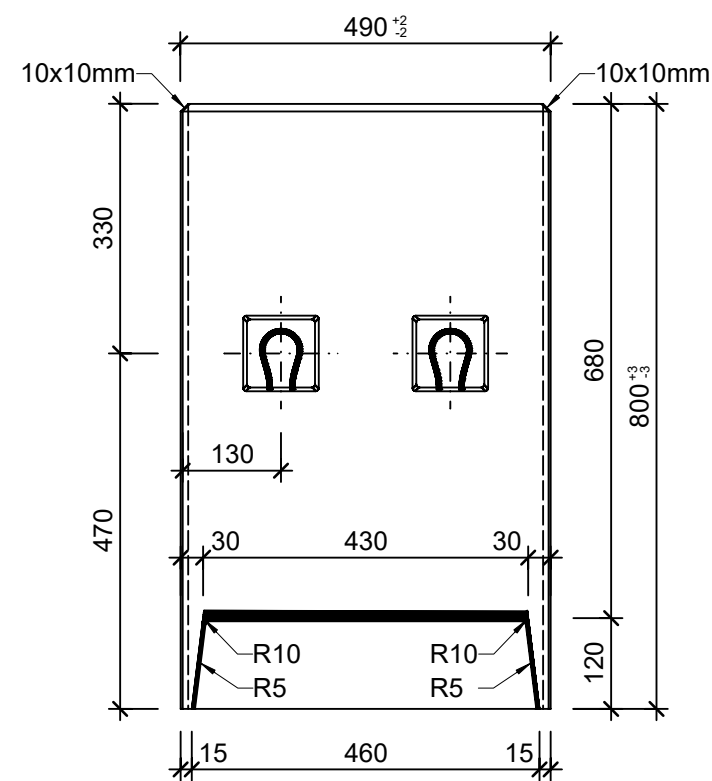
Ansicht 1-1, 1:10
