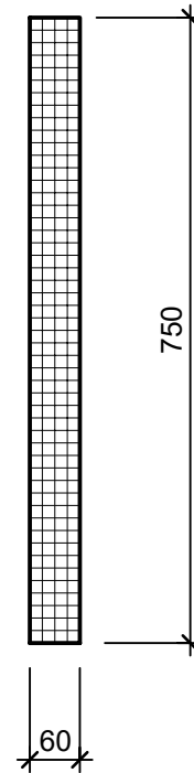
Schnitt 2-2 1:10
