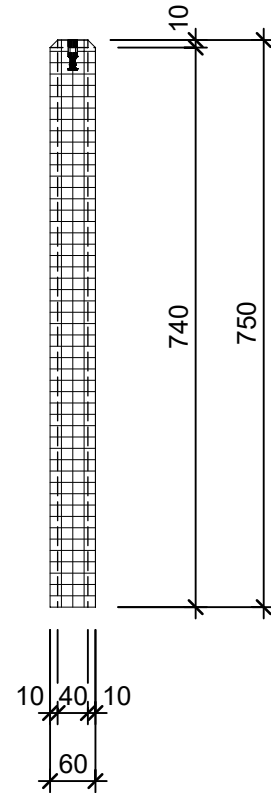
Schnitt 2-2 1:10
